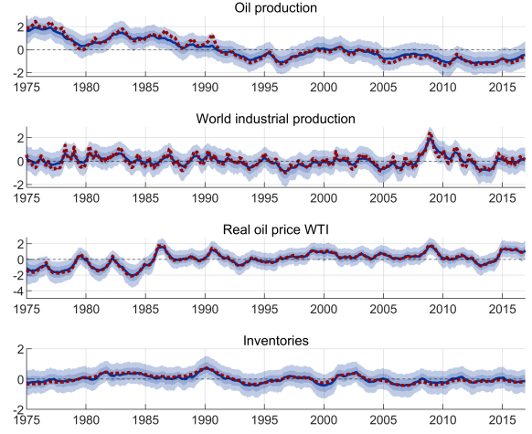
(b) SV-t
