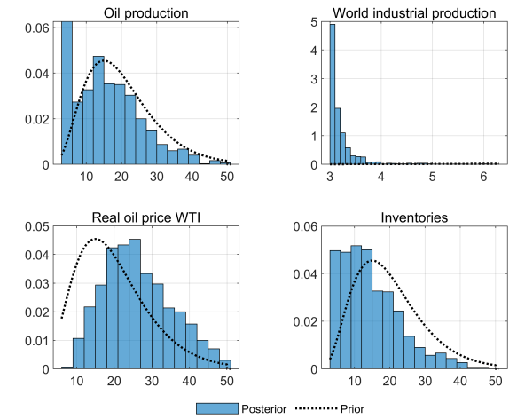
(b) SV-t
