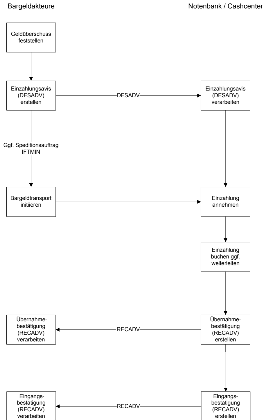
Prozessdiagramm EANCOM-Nachrichten Einzahlung (DESADV / RECADV)
